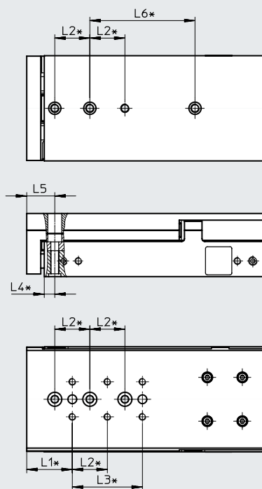
DGST-12-50/80
