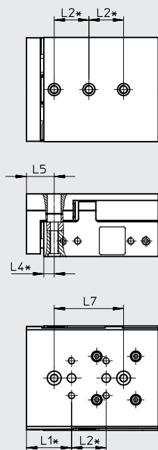
DGST-12-20
